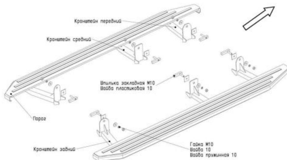
Рис. 1 Схема установки комплекта порогов
